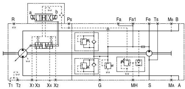
回路图
