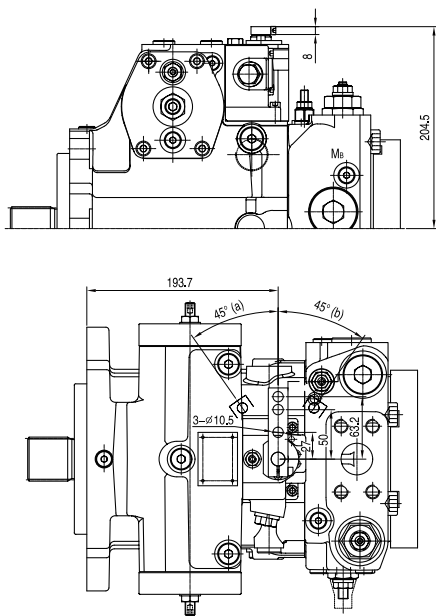
液压控制，机械伺服，HW
