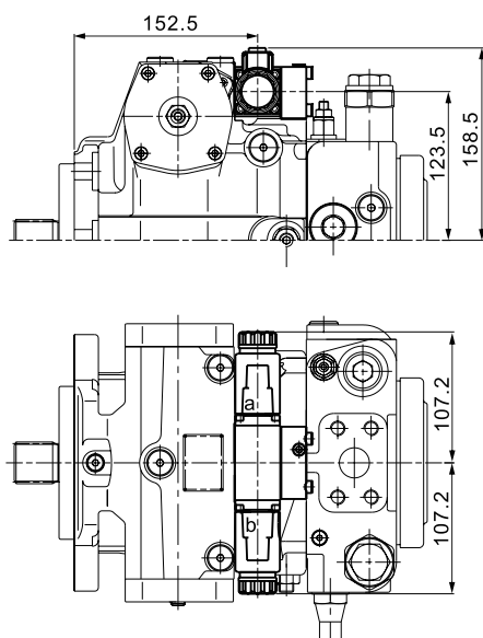
电气控制，带比例电磁铁，EP
