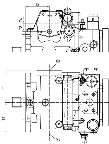
外形图
