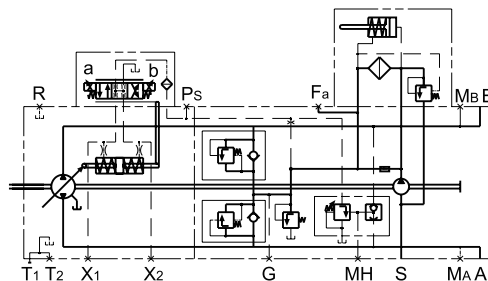
原理图
