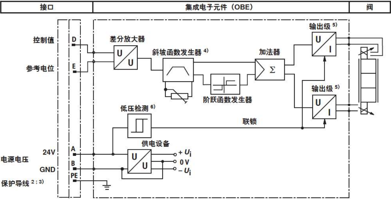
电路图/连接分配
